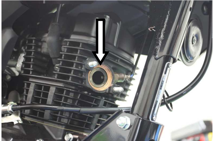
Verificare che la guarnizione sia correttamente posizionata nella rispettiva sede Check that the OE gasket is correctly placed in its seat
