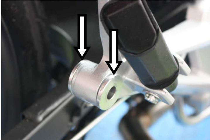
Sostituire nella pedana passeggero DX il Silent Block con gli spessori forniti On the RH passenger footrest, replace silent block with spacers given in the fitting kit
